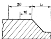
Рис.8.1. Кромка литой детали
